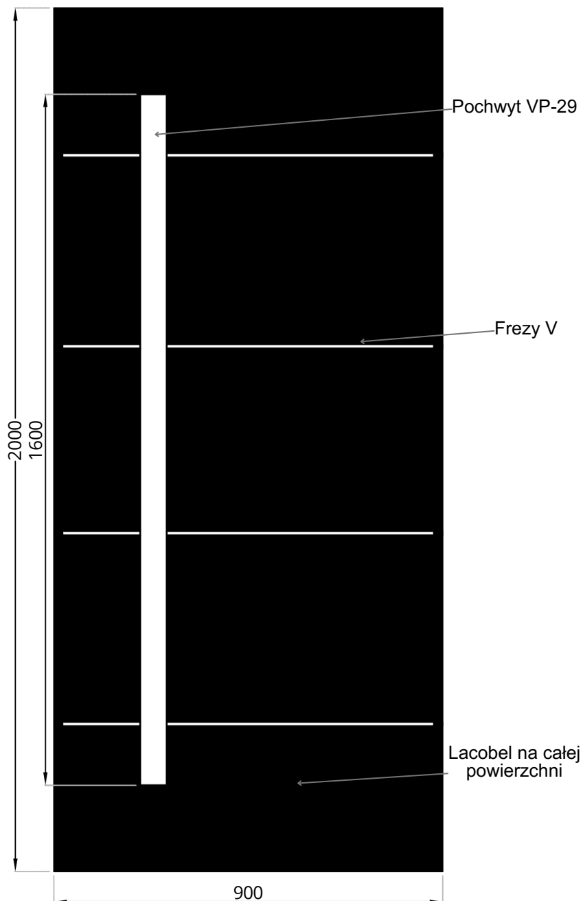
WIDOK OD STRONY ZEWN.
